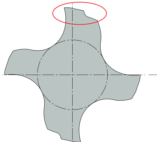
Regulärer Fräsertyp
